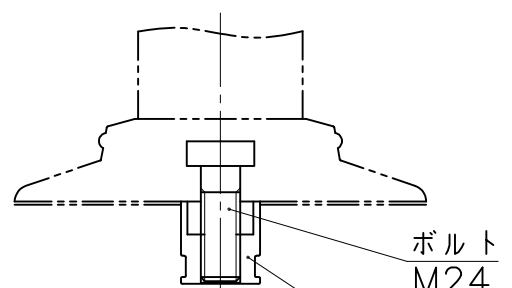
埋設用脚セット図
